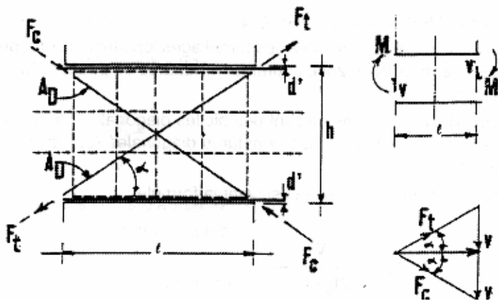
Fig.7.12 : Efforts dans les bielles du linteau
