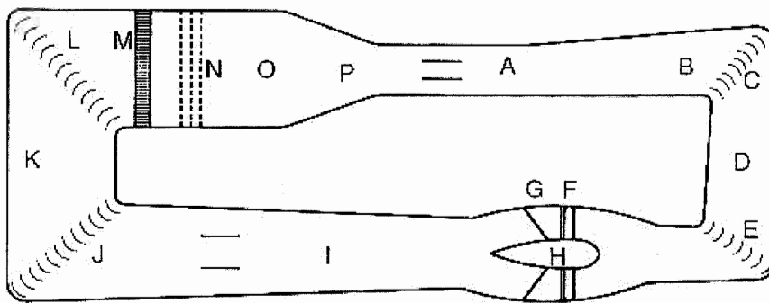
A : veine d'essais – B : diffuseur – D, I, K : retour diffuseur – C, E, J, L : aubes de guidage F : hélice – H, G : nacelle moteur et supports – M : nids d'abeilles – N : filets métalliques O : chambre de tranquillisation – P : convergent.
