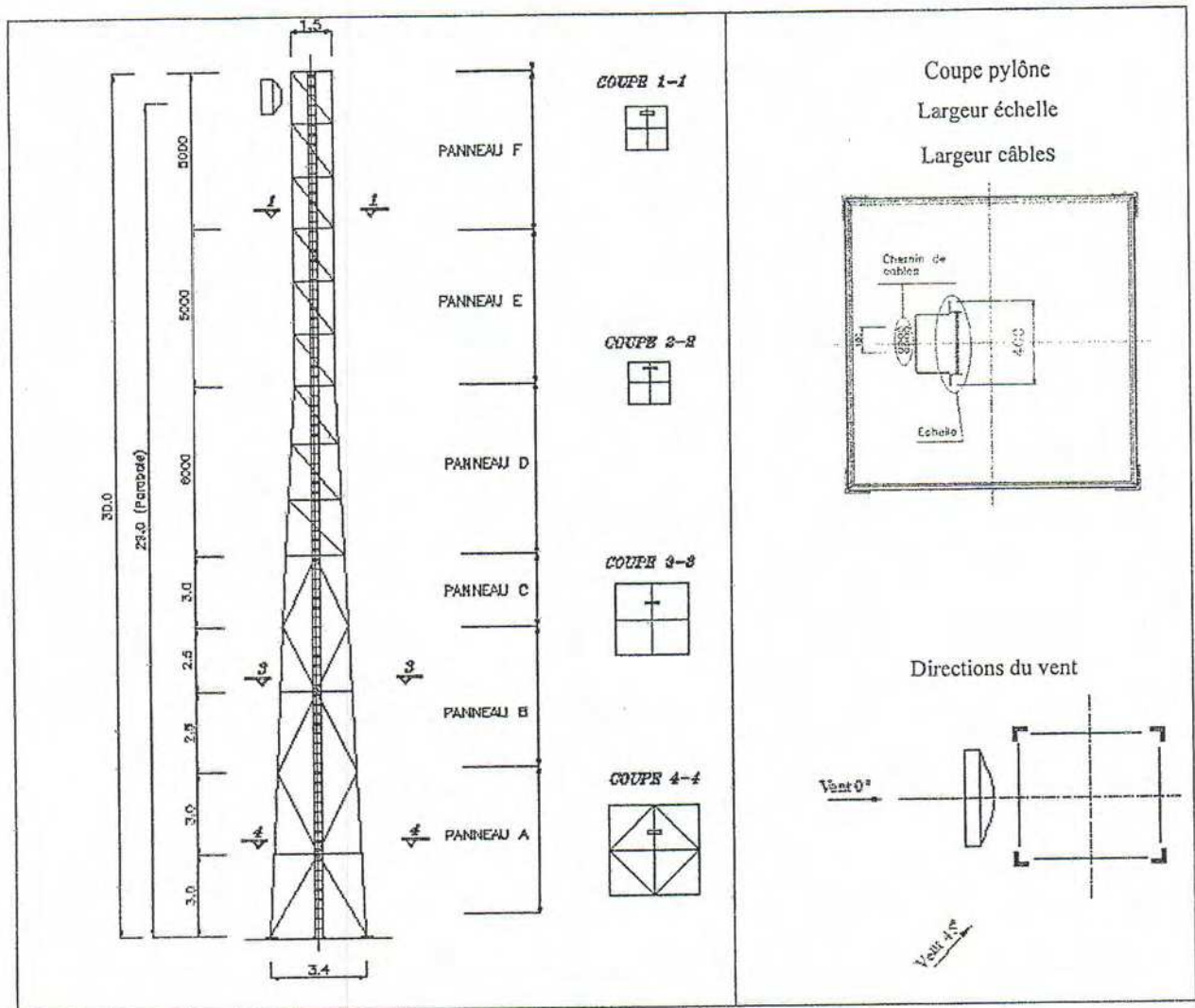
Figure 8 : Structure en treillis de type pylône
