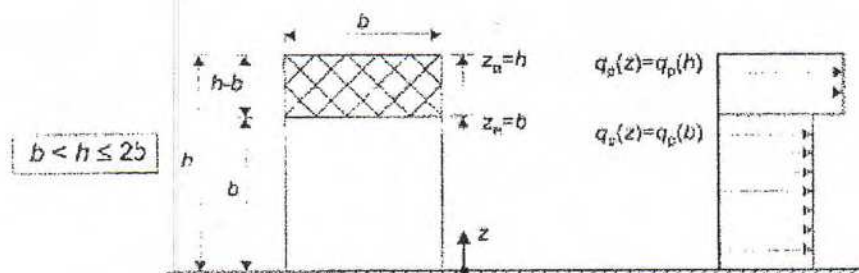
Figure 1 : Subdivision du bâtiment pour la définition de la hauteur de référence
