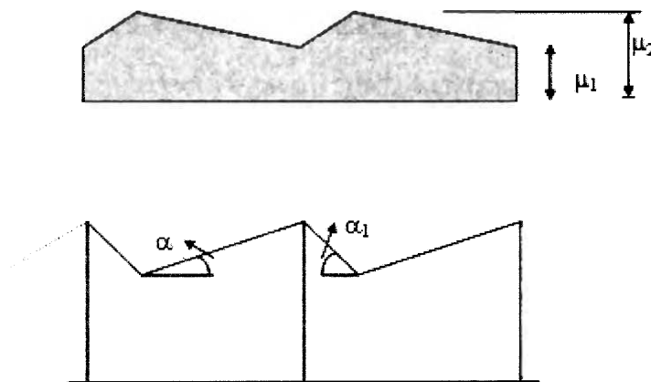
Figure 10 : Coefficient de forme des toitures à redans
