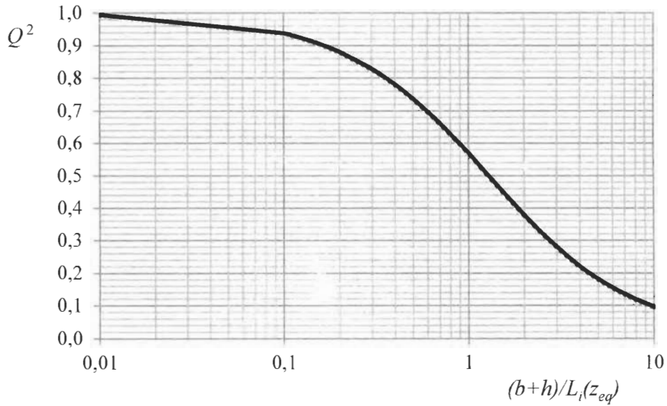
Figure 3.2 : Valeurs de la partie quasi statique ( Q^2 )
