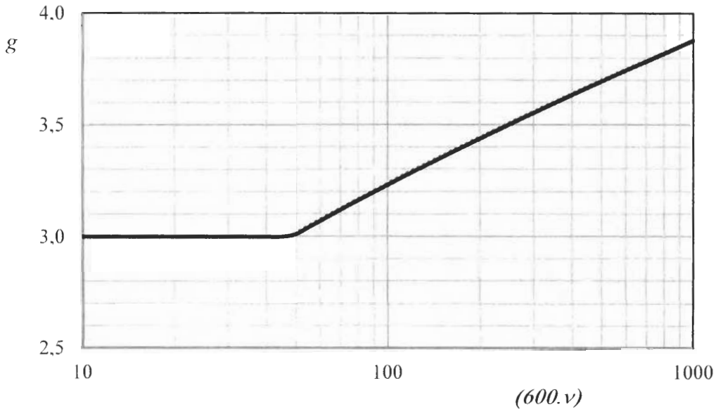
Figure 3.5 : Facteur de pointe
