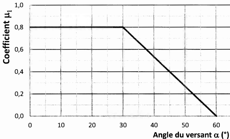
Figure 7 : Coefficients de forme - Toitures à deux versants
