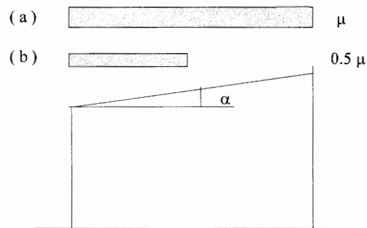
Figure 4 : Coefficient de forme - toitures à un versant
